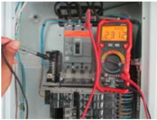
Pic:7 มีการวัดแรงดันไฟฟ้า เฟสที่ 3 พบว่าแรงดันไฟฟ้าปกติ
